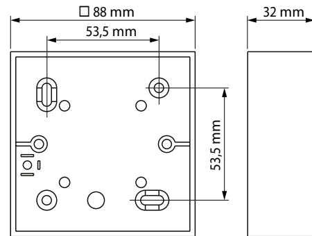
Puszka montażowa do montażu natynkowego
